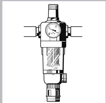
Waterfilter FK74C 3/4" met reduceerventiel voor het instellen van de uitgaande waterdruk
